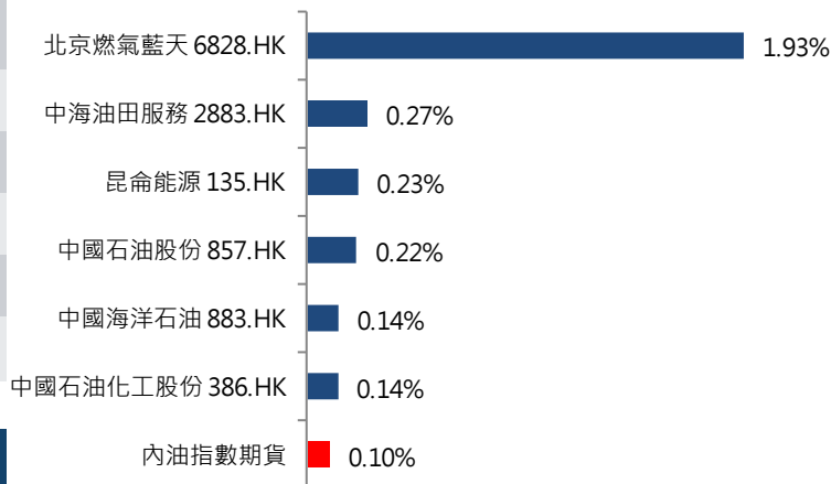
每五分鐘平均買賣差價比較 (2018年9月28日)
